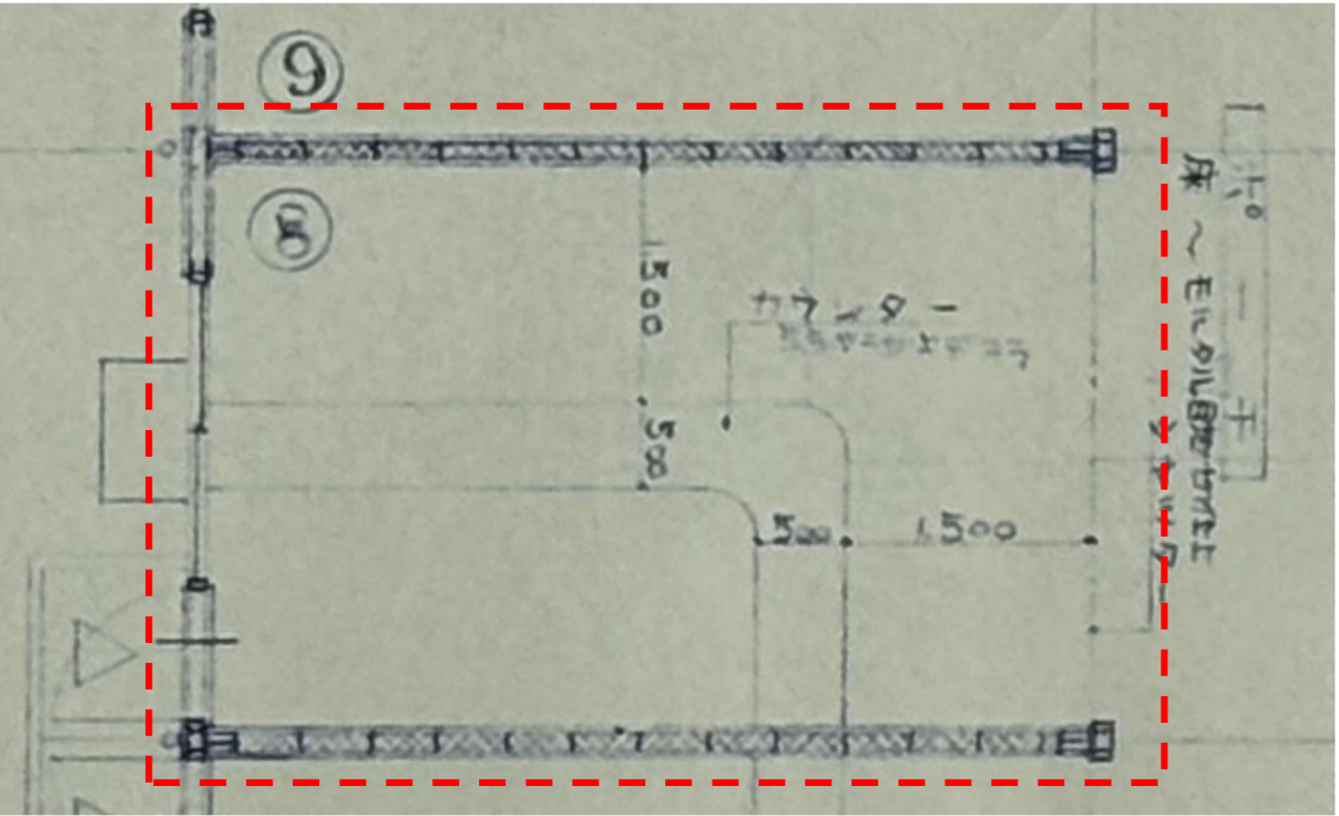
④平面図 （縦 3.6m × 横 5.4m = 19.44 m 2 ）
